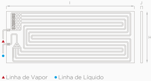
Equipamento: Painel Solar Termodinâmico X6 | X12 | X16 | X32
