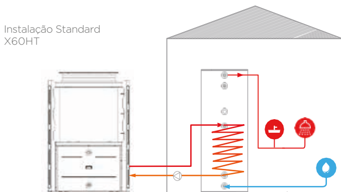
Instalação com Inércia X60HT (zonas climáticas frias)
