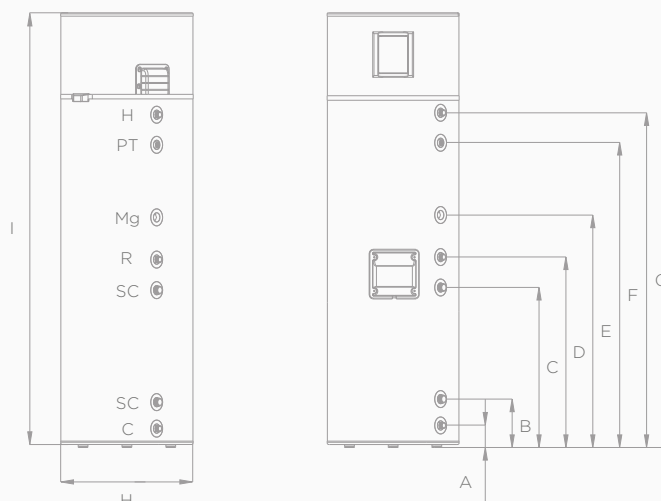
Impianto: Scaldabagno
