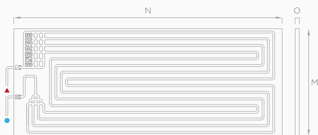
Impianto: Pannello Solare Termodinamico
