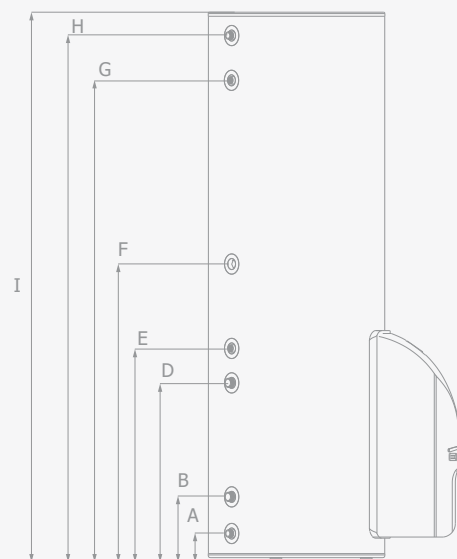
Raccords arrières: 5001 / 5001X
