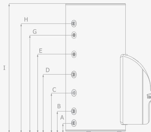
Raccords arrières: 3001 / 3001X
