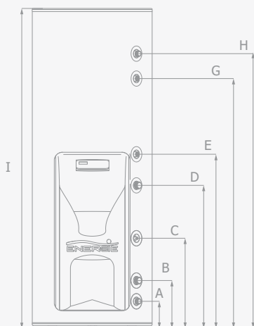
Raccords frontaux: 2001 / 2001X | 2501 / 2501X
