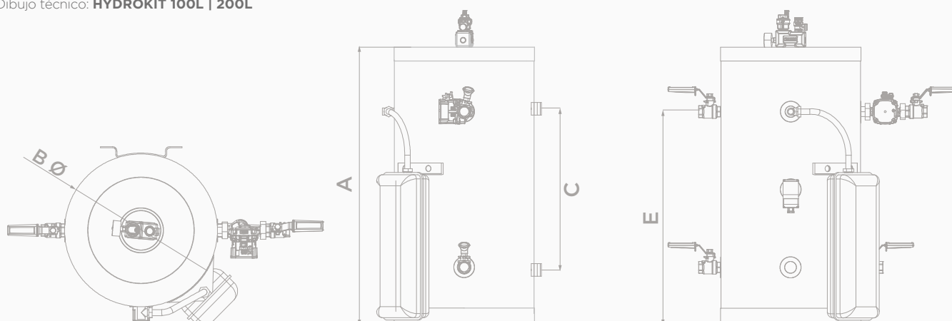
Dibujo técnico: HYDROKIT 100L | 200L
