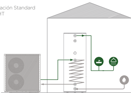
Instalación Standard X75HT
