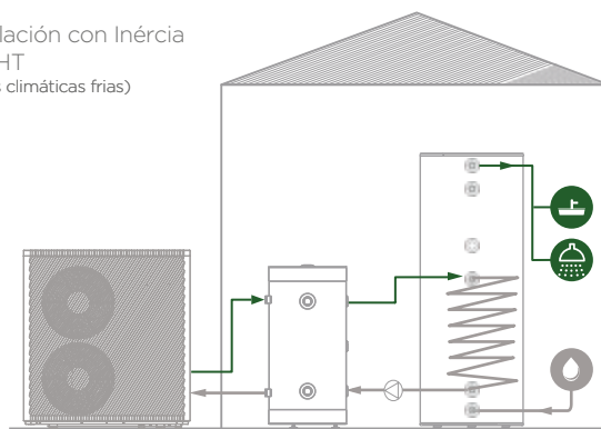
Instalación con Inercia X60HT (zonas climáticas frías)
